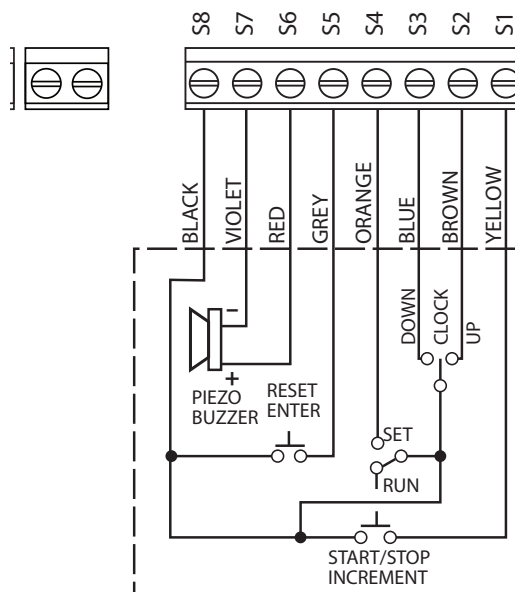
ATSTCS Wiring Diagram
